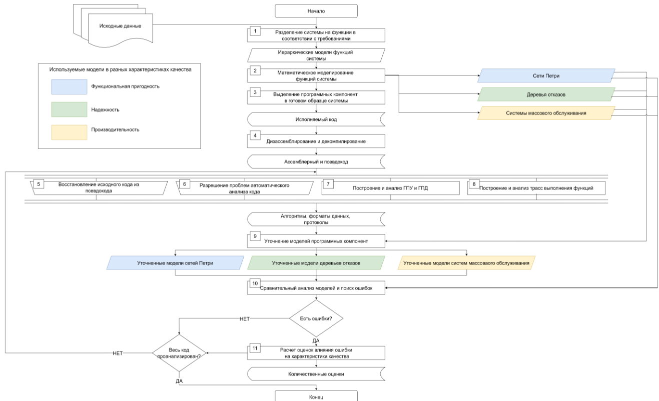
Рисунок 2 – Блок-схема алгоритма поиска ошибок
