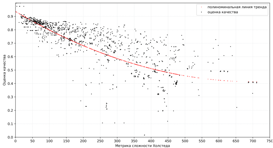
Рисунок 7 – Зависимость качества КЭ СУ от сложности ПО
