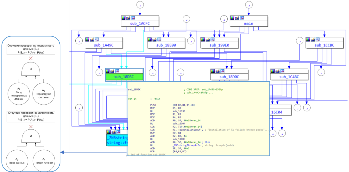
Рисунок 5 – Анализ исполняемого кода функции «обновление ПО»
